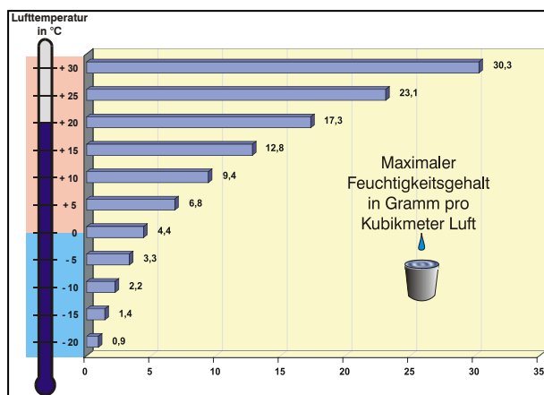
Maximaler Wasserdampfgehalt (= 100 % relative Luftfeuchte) in Gramm pro m 3 Luft bei verschiedenen Temperaturen.
